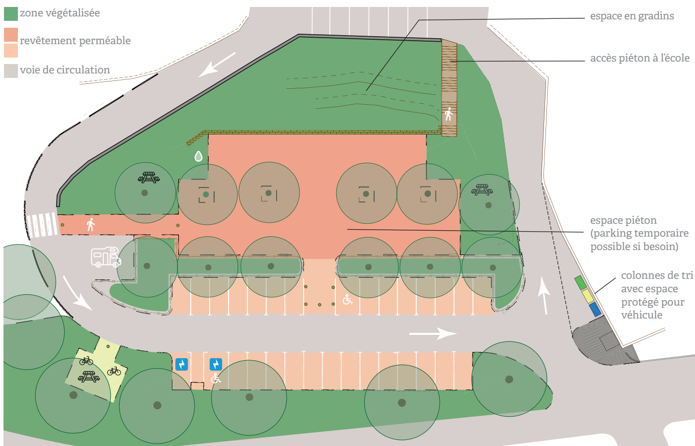
Schémas de principe
